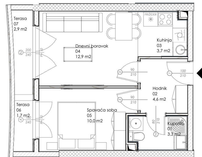
ORGANIZACIJA STANA L1-I-J3
